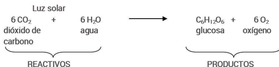
Fig. 4. Ecuación química que representa el fenómeno de la fotosíntesis
