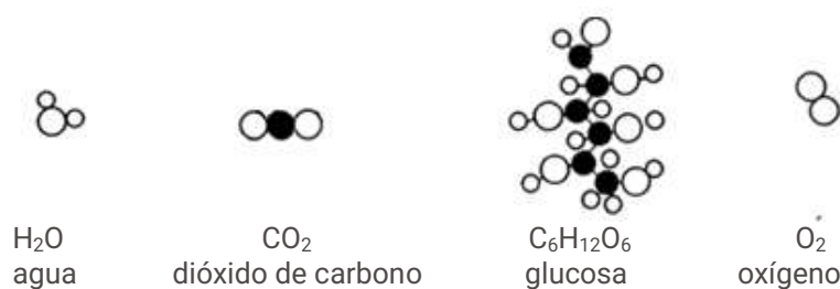
Fig. 3.: representación esquemática con modelo de esferas y de la fórmula molecular de las moléculas de los compuestos que intervienen en el proceso de fotosíntesis
