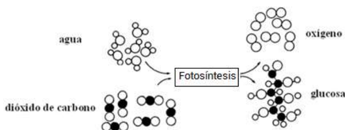
Fig. 5: Modelo esquemático que representa el fenómeno de la fotosíntesis
