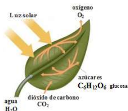
Fig. 1. Representación gráfica del proceso de fotosíntesis en una hoja [2].
